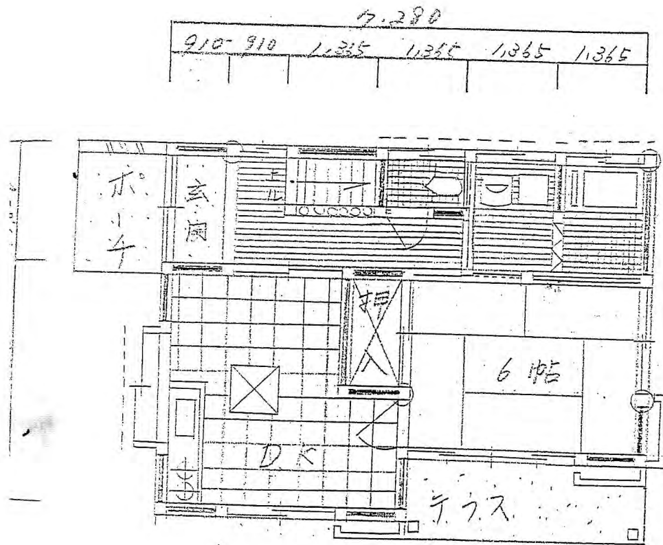
1階平面図 11坪
